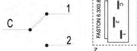
Schema elettrico Wiring diagram
