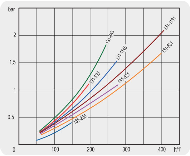
PERDITE DI CARICO (32 cSt) PRESSURE DROP (32 cSt)
