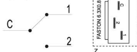
Schema elettrico Wiring diagram
